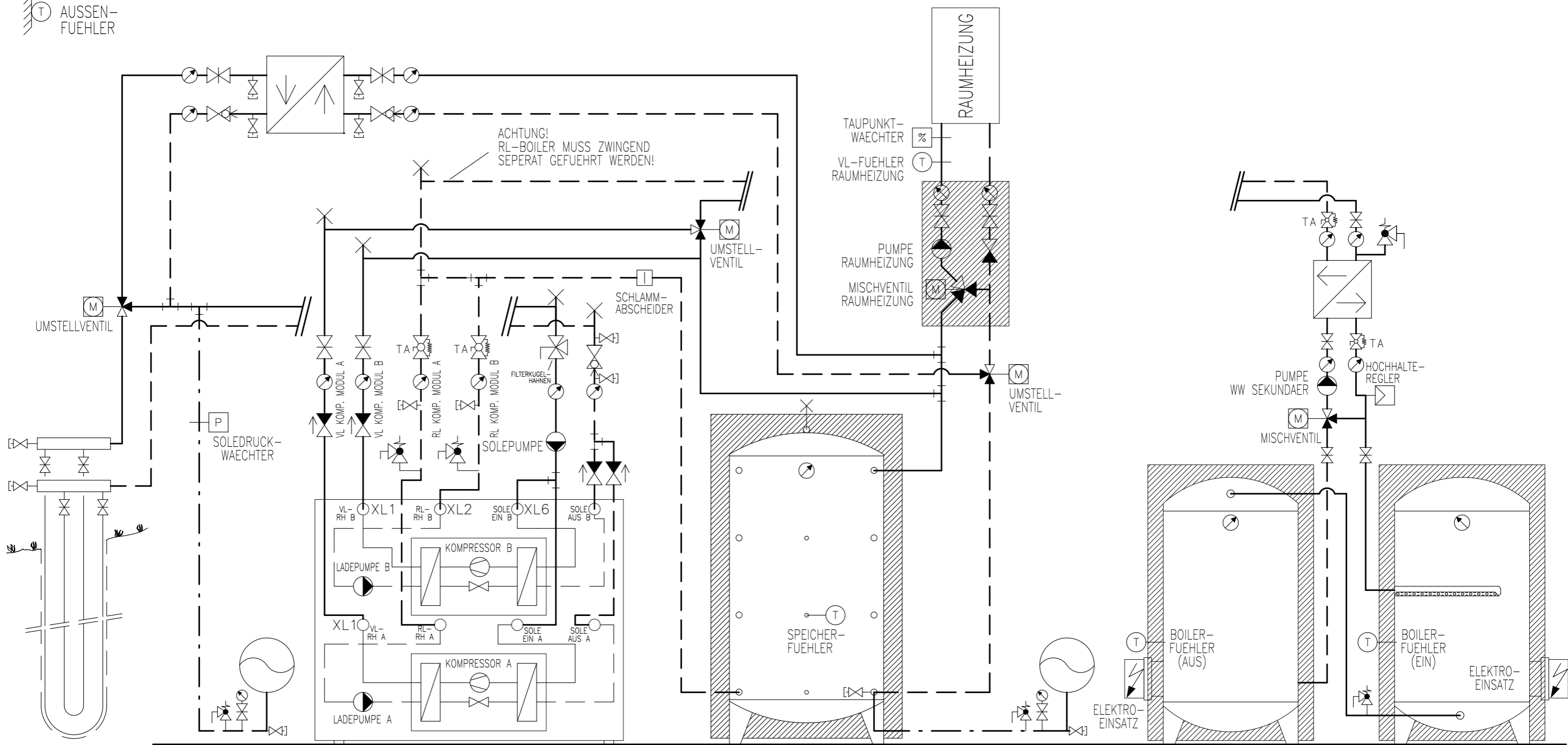
ERDSONDE EXP.-GEFAESS WAERMEPUMPE NIBE F1345-... (FRONTANSICHT) HINWEIS: DIE SOLEPUMPE IST NUR BEI DER 1345-40/-60 EXTERN. BEI DEN ANDER 1345-/1355- SIND DIESE INTERN. SPEICHER EXP.-GEFAESS BOILER 2 BOILER 1
