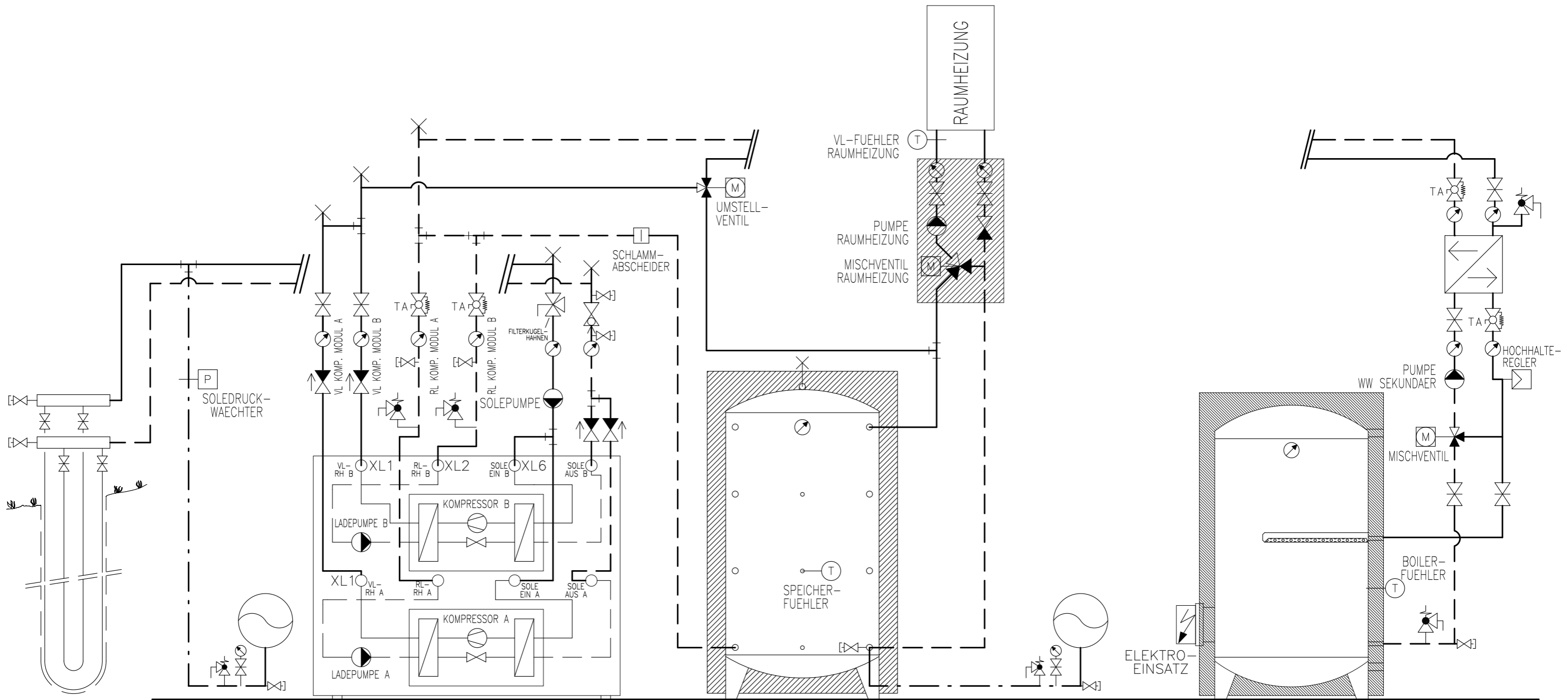
ERDSONDE EXP.-GEFAESS
