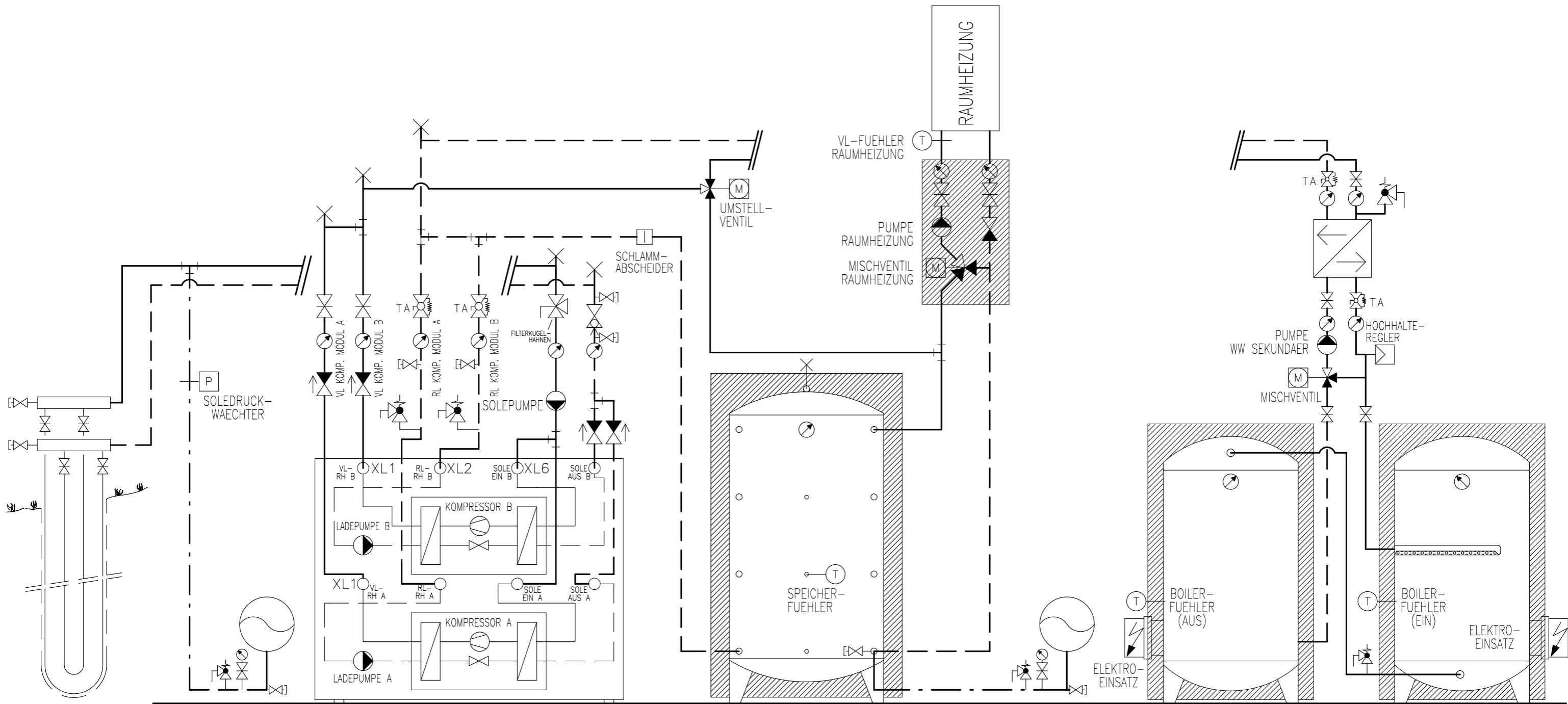
ERDSONDE EXP.-GEFAESS WAERMEPUMPE NIBE F1345-... (FRONTANSICHT) HINWEIS: DIE SOLEPUMPE IST NUR BEI DER 1345-40/-60 EXTERN. BEI DEN ANDER 1345-/1355- SIND DIESE INTERN. SPEICHER EXP.-GEFAESS BOILER 2 BOILER 1
