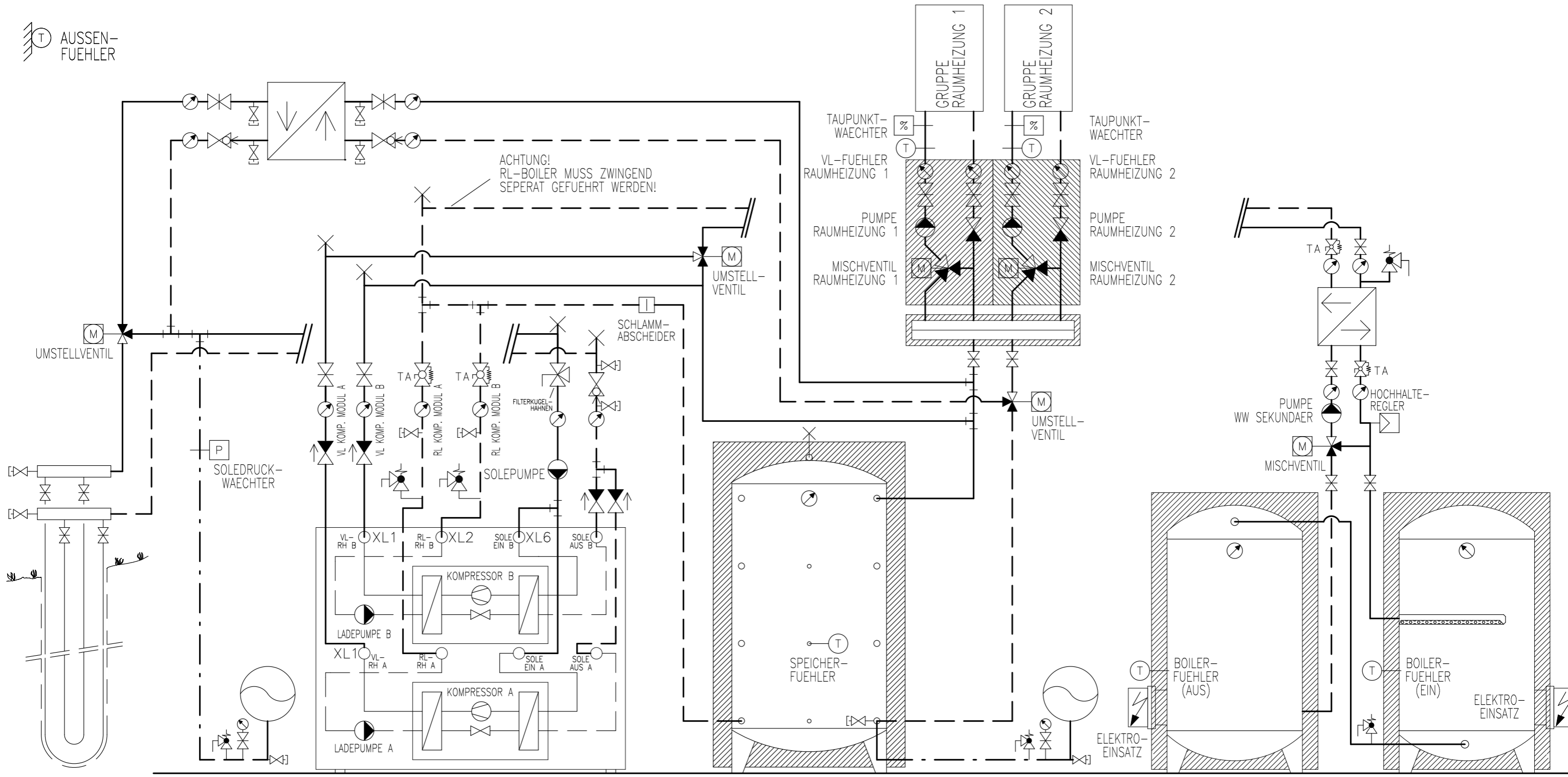
ERDSONDE EXP.-GEFAESS WAERMPUMPE NIBE F1345-... (FRONTANSICHT) HINWEIS DIE SOLEPUMPE IST NUR BEI DER 1345-40/-60 EXTERN. BEI DEN ANDER 1345-/1355- SIND DIESE INTERN SPEICHER EXP.-GEFAESS BOILER 2 BOILER 1
