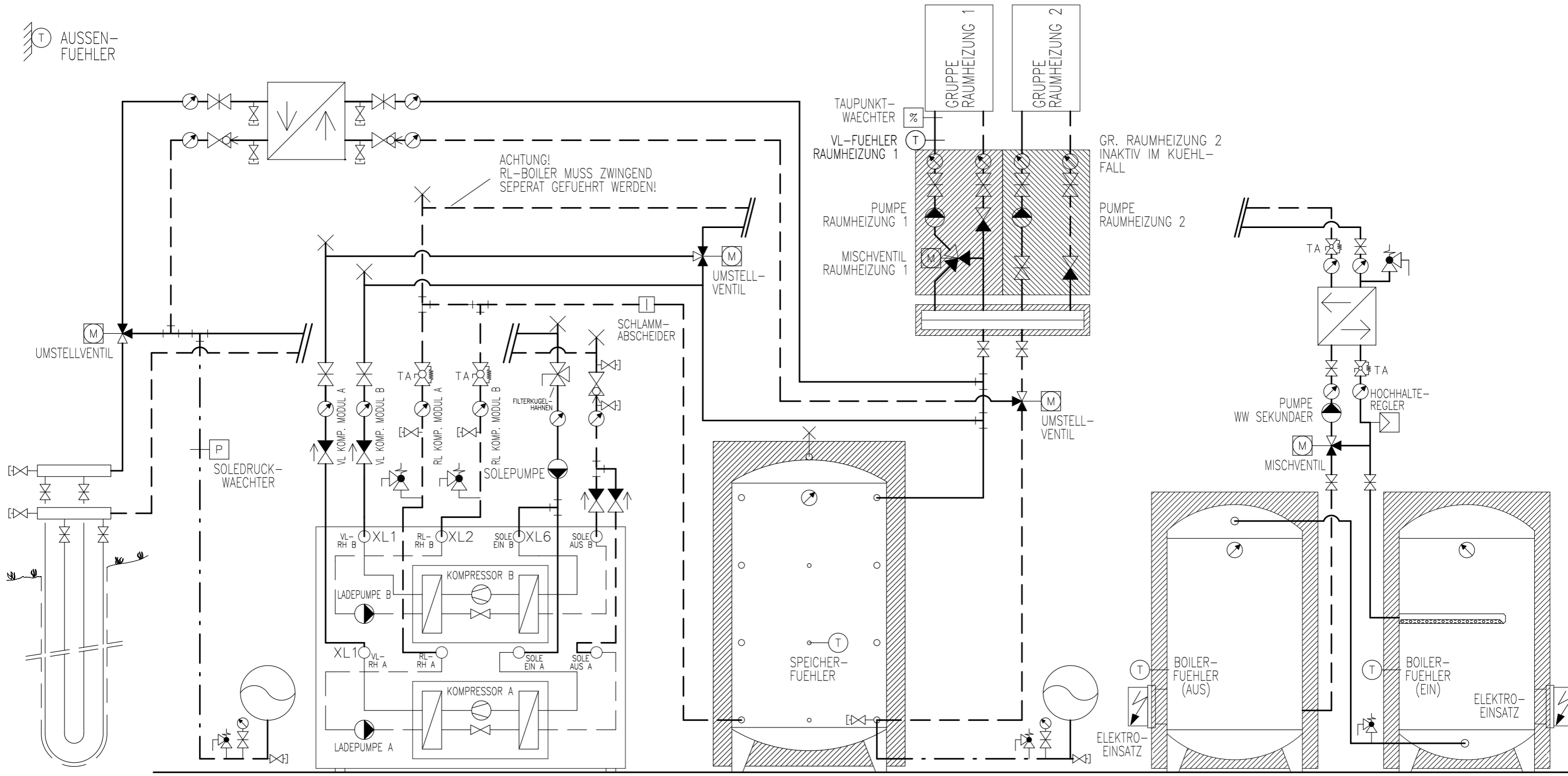
ERDSONDE EXP.-GEFAESS WAERMEPUMPE NIBE F1345-... (FRONTANSICHT) HINWEIS: DIE SOLEPUMPE IST NUR BEI DER 1345-40/-60 EXTERN. BEI DEN ANDER 1345-/1355- SIND DIESE INTERN. SPEICHER EXP.-GEFAESS BOILER 2 BOILER 1
